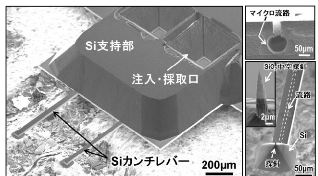
図：中空構造を有するナノニードル搭載型バイオプローブ（単一細胞ナノ加工・計測用ツール）
