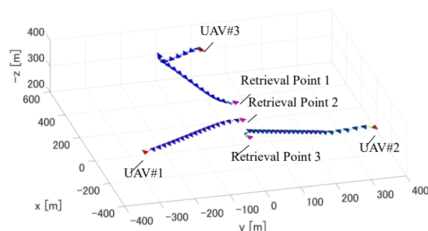
図1. 最適タスクアサインと3次元最適軌道の例
