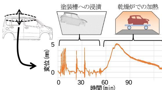
Fig.2 測定例(ルーフパネル上下動)
