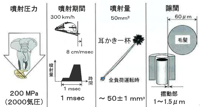
図3. 高压喷射のスケールイメージ
